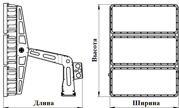
Габаритные размеры
